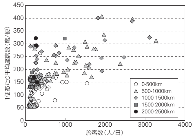
■図四 距離帯別の旅客数と機材サイズ(日本2004)
