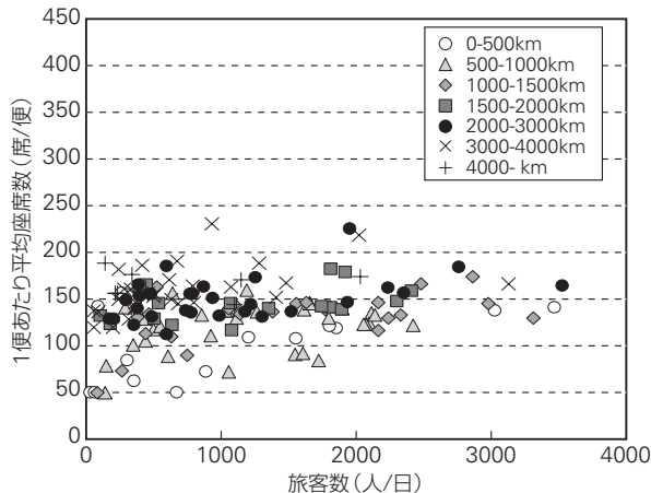
■図三 距離帯別の旅客数と機材サイズ(米国2004)
