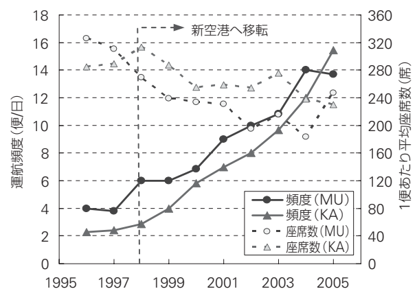
■図—8 複数エアラインによる頻度競争の例(上海路線)
