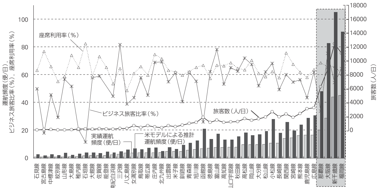
■図—5 米国市場に対する回帰モデルの羽田路線への適用結果
