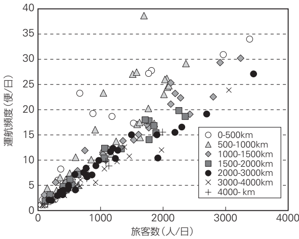
■図一 距離帯別の旅客数と運航頻度(米国2004)
