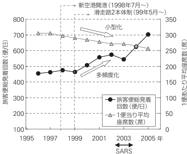
■図—6 香港国際空港における頻度、機材サイズの変化
