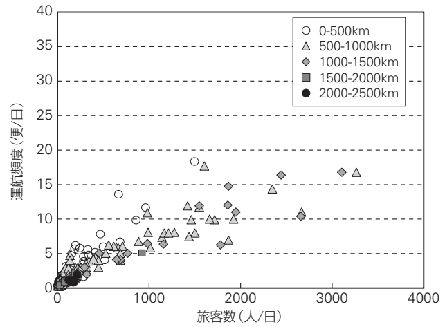
■図二 距離帯別の旅客数と運航頻度(日本2004)
