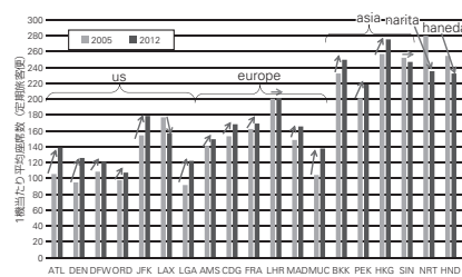
■図—1 世界の主要空港の1便当たり平均座席数(定期旅客便)
