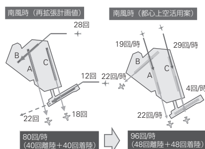
■図一3 都心上空活用による容量拡大方策
