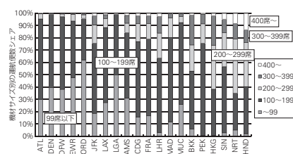
■図—2 世界の主要空港の機材サイズ別の運航便数シェア(定期旅客便)(2012)
